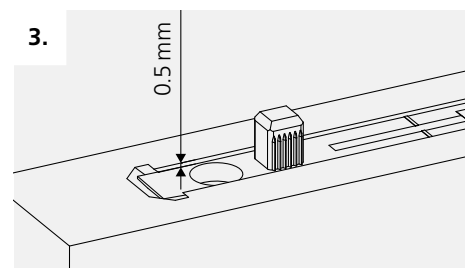
3. Optimale diepte verzonken verbinder = 0.5 mm
